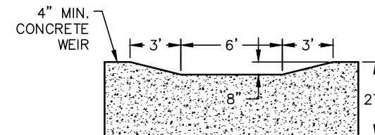
E OVERFLOW WEIR SECTION N.T.S.
